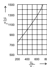
Schaltspannungsdiagramm Arc Voltage-Diagram
